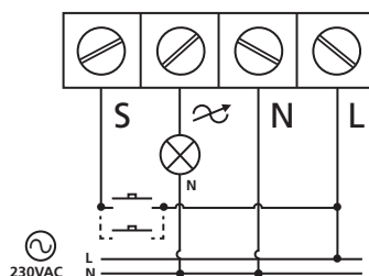
Schéma de montage
