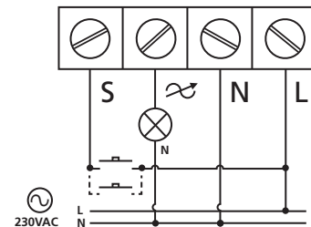
Kopplingsschema
