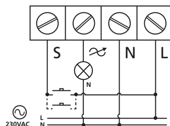
Kytkeyntäkaavio
