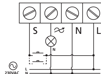
Aansluitschema
