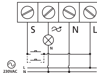
Wiring scheme
