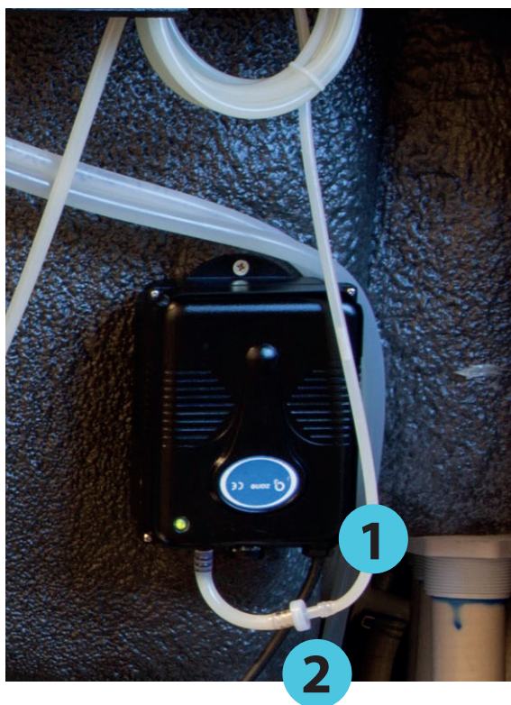
1 - Ozonslang 2 - Backventil
