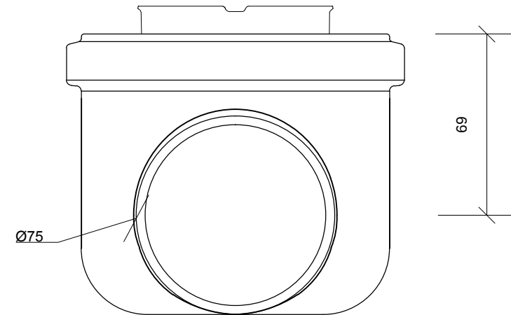
Front Opstalt/Front Elevation/Frontansicht
