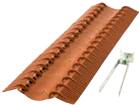
Decra nockband och nockbeslag För tätning och ventilation av nock. Nockbeslaget är justerbart i höjdlöd.
