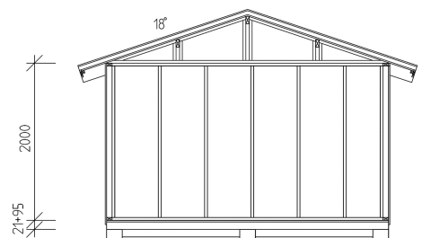
Sektion
