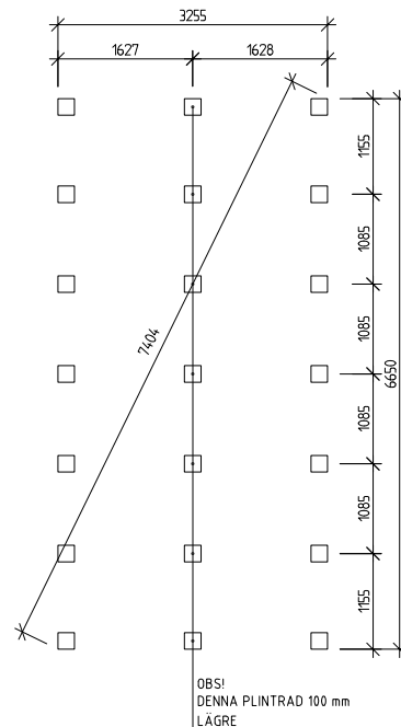
Plintritning
