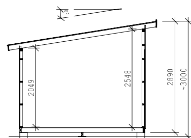
SEKTION
