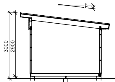
Sektion
