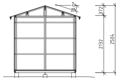
Sektion
