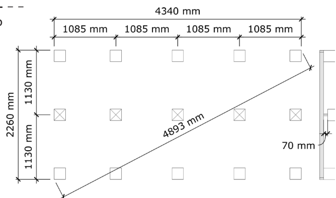
Plinritning
