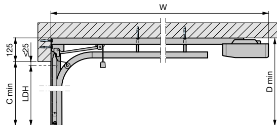
Vertikalsnitt
