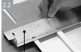
Kopfprofil Rückwand top frame profile back wall profil de tête paroi arrière kopprofiel achterwand
