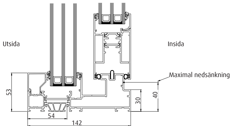
2-spårprofil för skjutbart system med Köldbryggebrytning.
