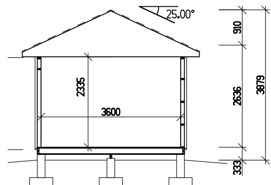
Sektion
