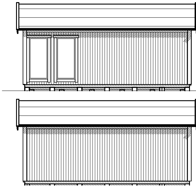
Långsida
